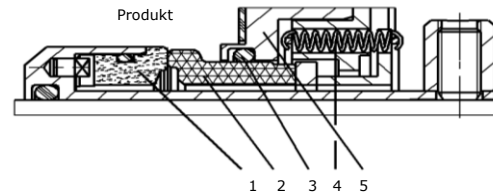
Enkel tätning
