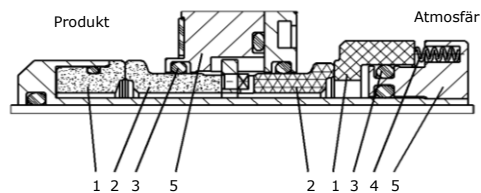
Dubbel tätning
